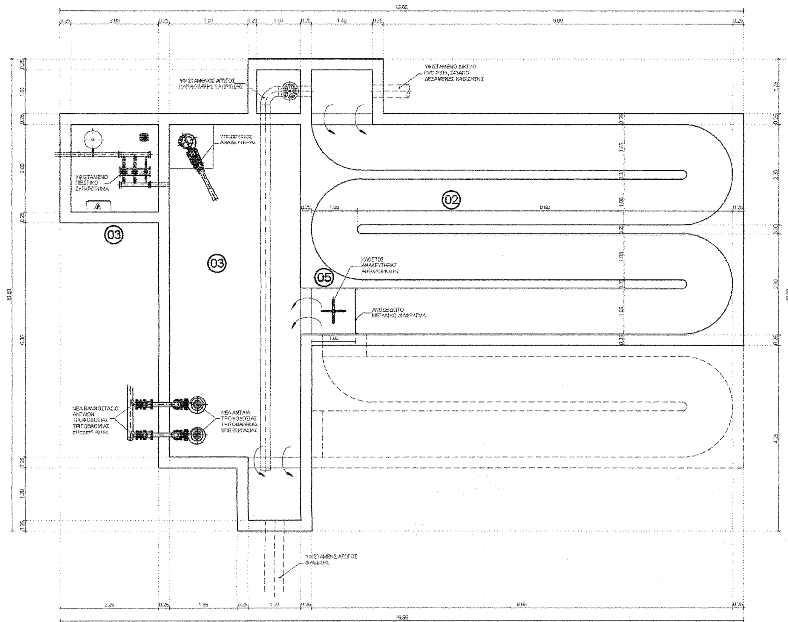
ΟΡΙΖΟΝΤΙΑ ΤΟΜΗ Α-Α
